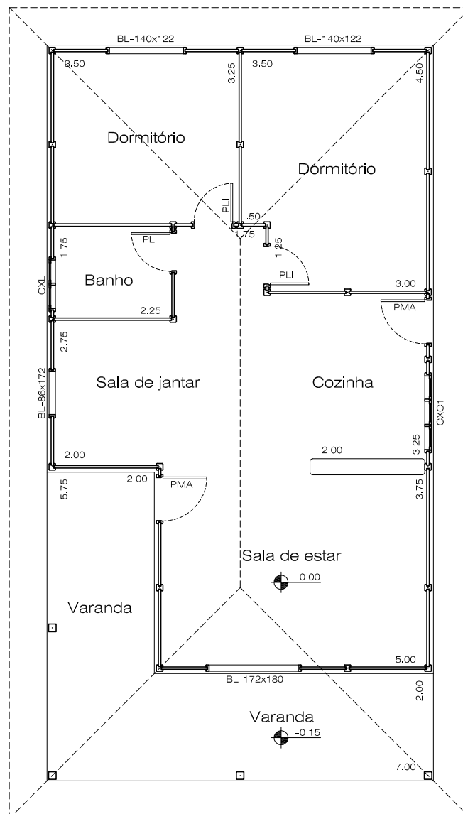
Planta baixa
