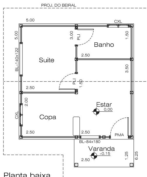
Planta baixa
