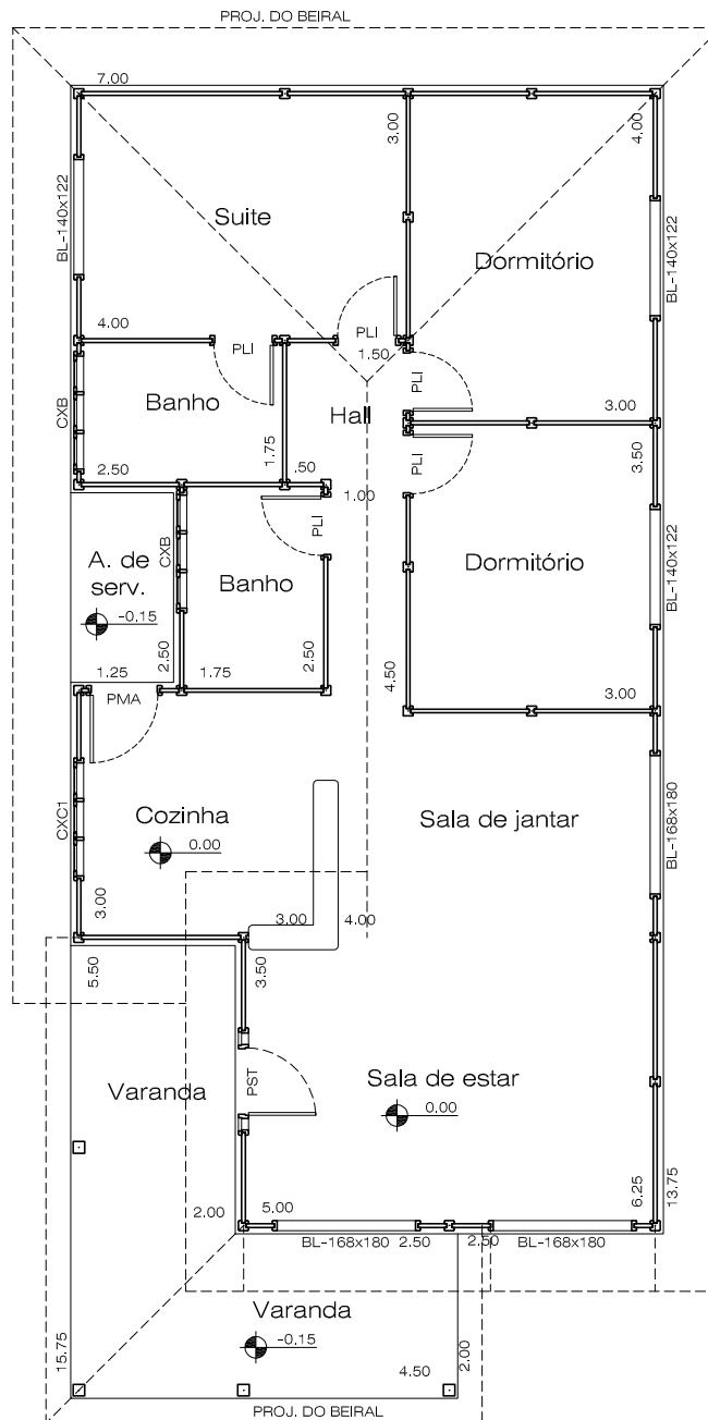
Planta baixa
