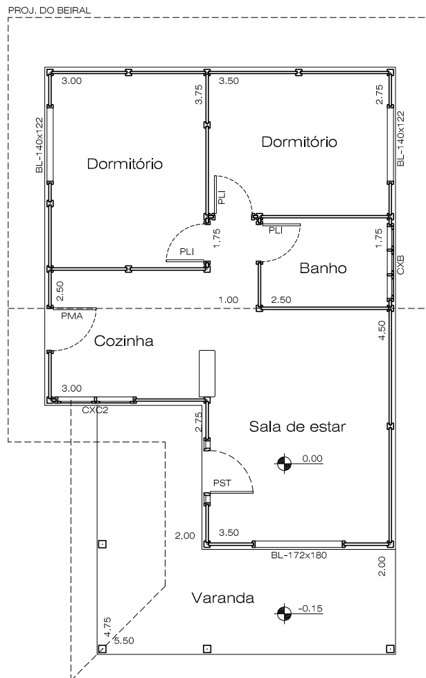
Planta baixa Obs.: - Medidas entre eixos Escala = 1:100
