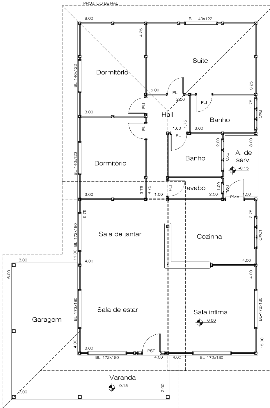
Planta baixa Obs.: - Medidas de eixo
