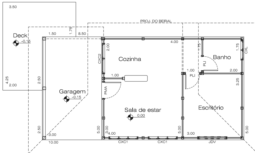
Planta baixa
