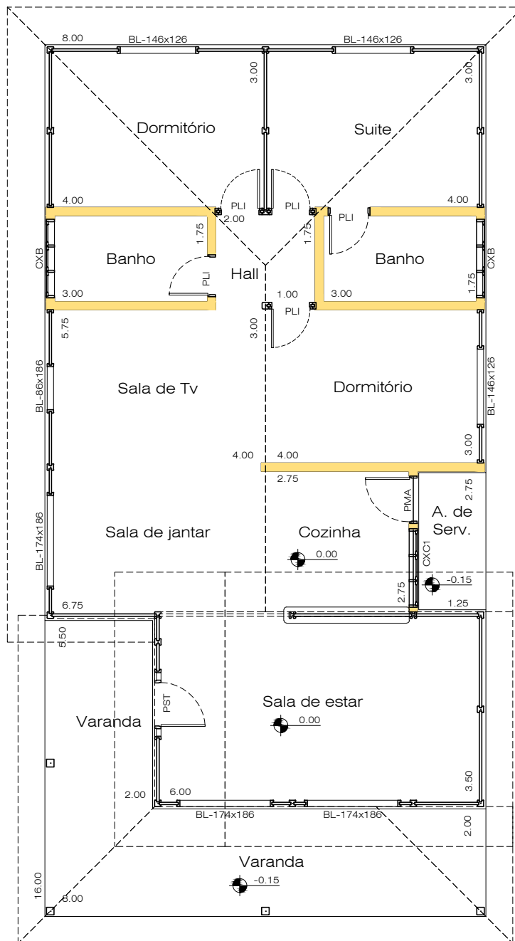
Planta baixa
