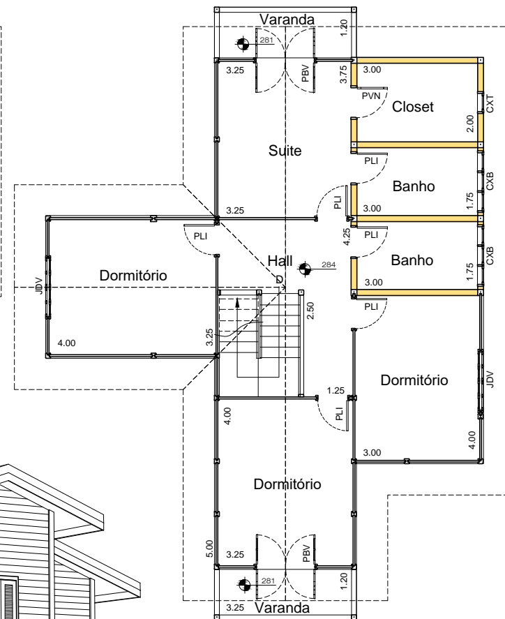
Planta baixa - Superior
